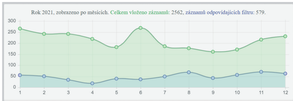
Graf 1: rizikové sexuální chování
