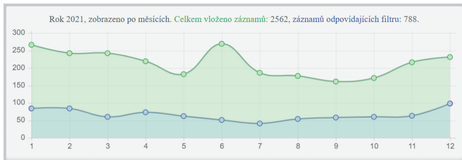
Graf 2: testování a místa, kde se mohou lidé nechat testovat na HIV
